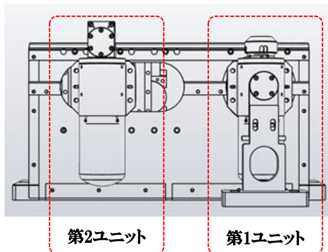
正面図
